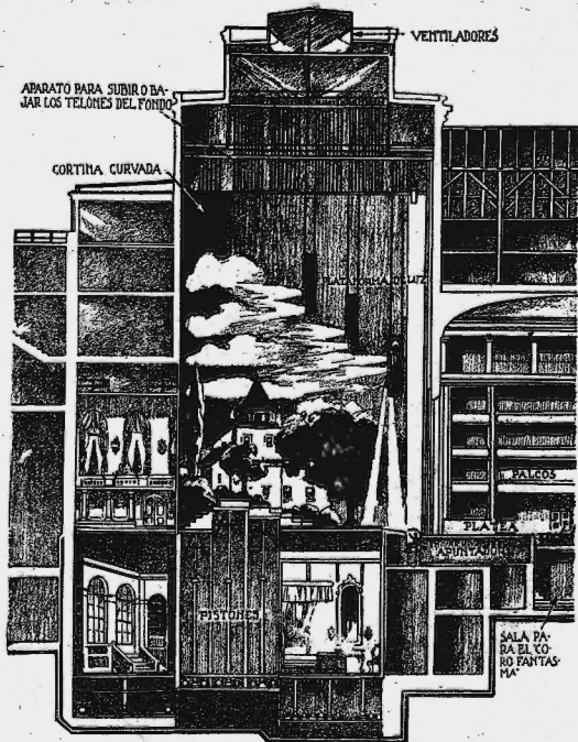
Dibujo seccional del escenario de un nuevo teatro alemán; decoraciones enteras pueden colocarse en posición sobre plataformas para rápidos cambios de escena, obteniéndose muchos efectos novedosos.
