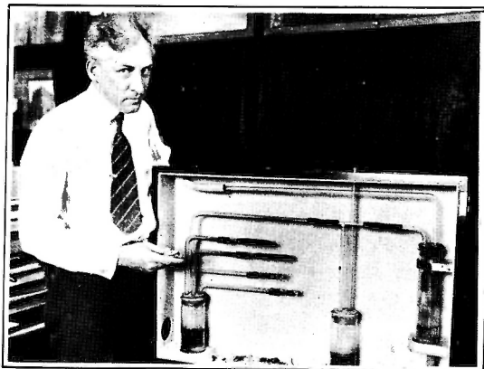
UN FUMADOR AUTOMÁTICO.—Este curioso aparato, que se utiliza en el Departamento de Agricultura de los Estados Unidos para realizar pruebas de tabacos, puede "fumarse" al mismo tiempo cuatro puros. En la foto aparece su inventor, F. L. Goll, estudiando cuidadosamente los residuos de la combustión de cuatro clases distintas de tabaco.
