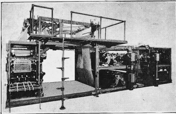
La nueva rotativa "Multicolor", construida especialmente para La Semana, por la casa Hoe.
